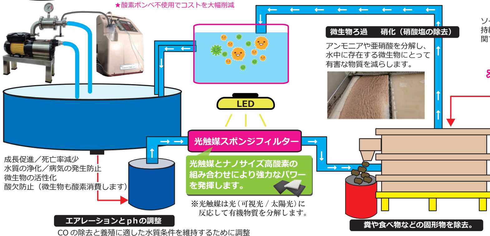
↓ ナノバブル発生装置
